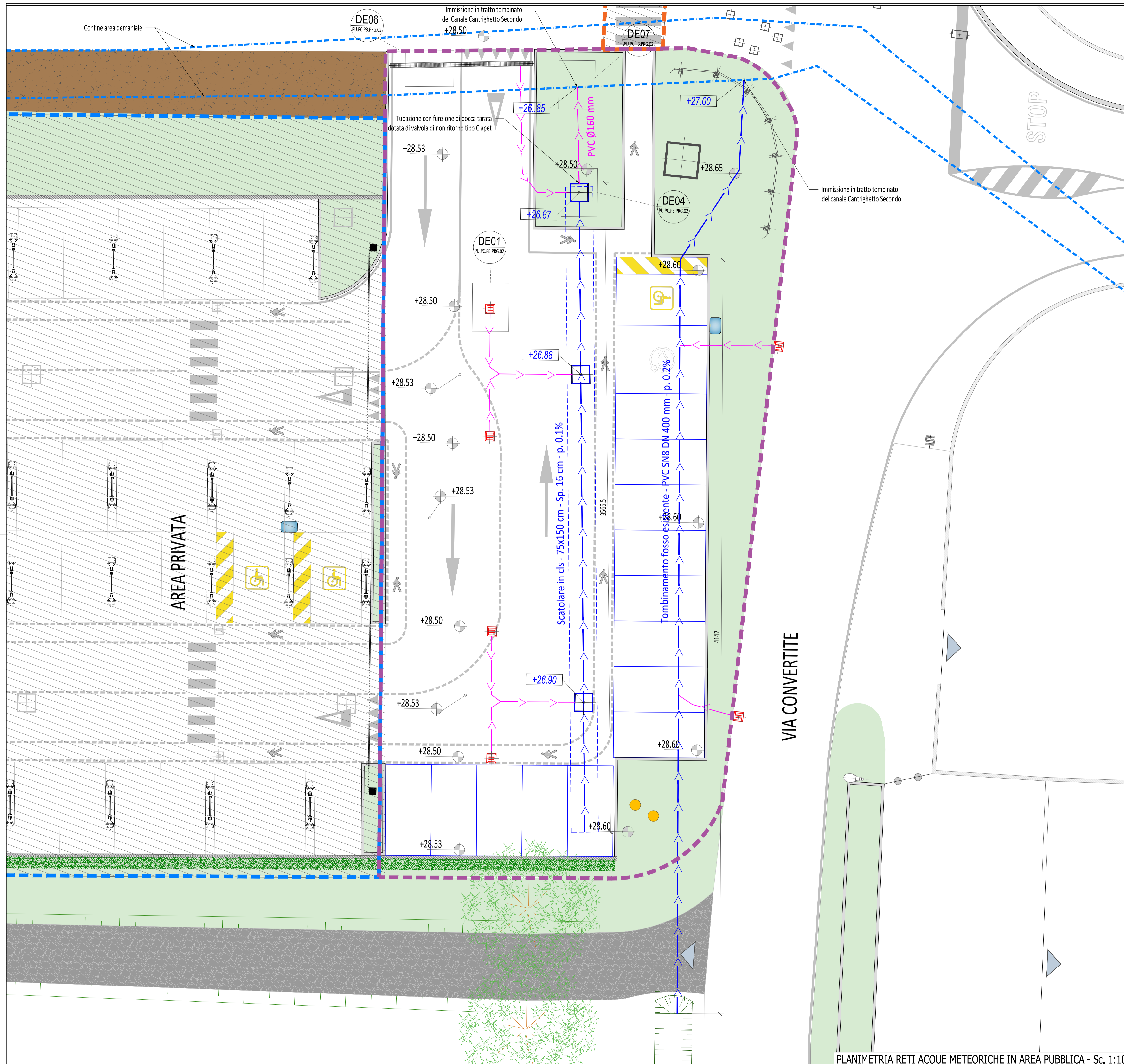
PLANIMETRIA RETI ACQUE METEORICHE IN AREA PUBBLICA - Sc. 1:100
